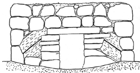
Plan och profilritning av myrjärnsblästa från Dalarna
